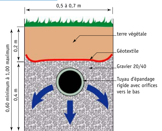
Coupe transversale
