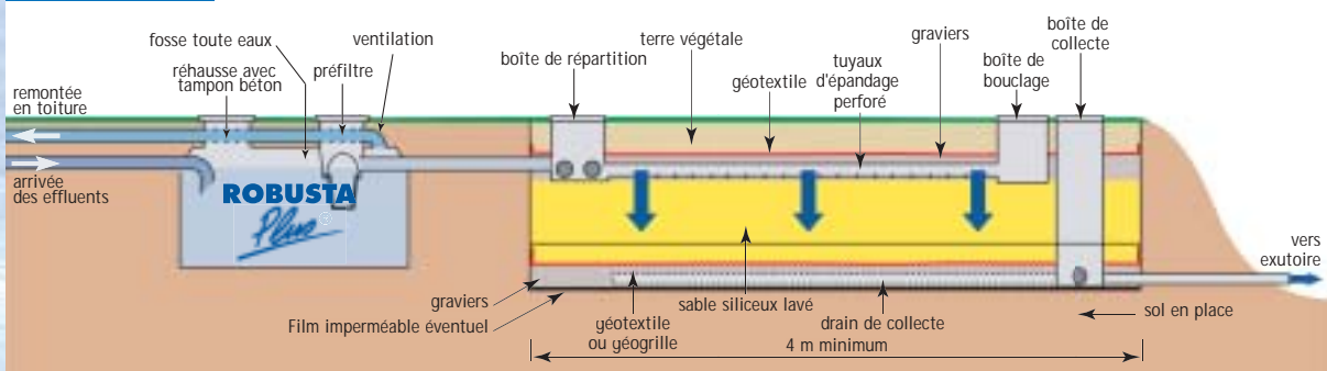
Coupe longitudinale
