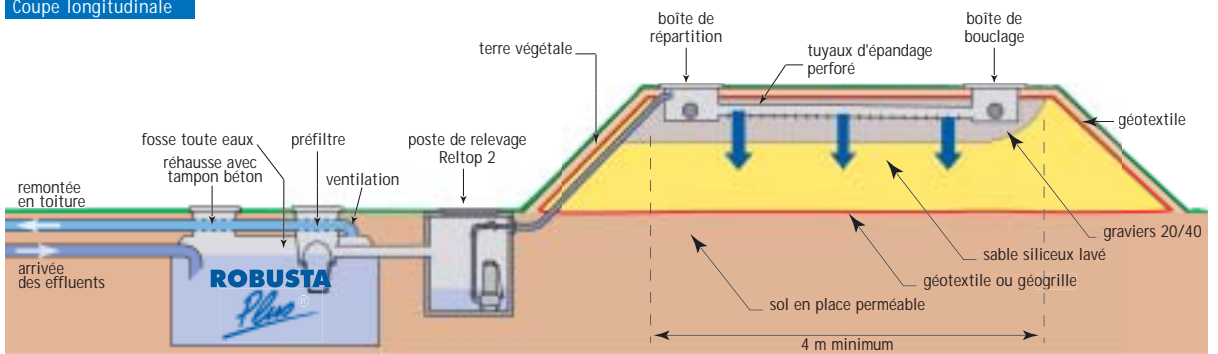
Coupe longitudinale
