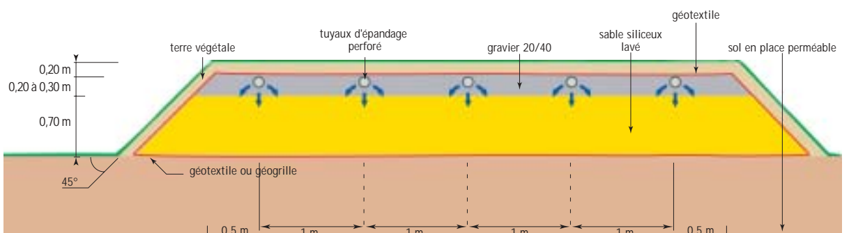
Coupe transversale
